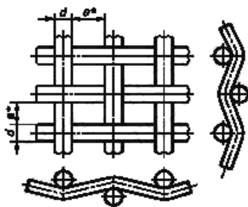
Рисунок 1 — Сетка типа СПП
