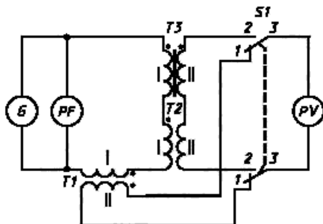
Рисунок 1 — Схема для измерений в динамическом режиме перемagnetизации
