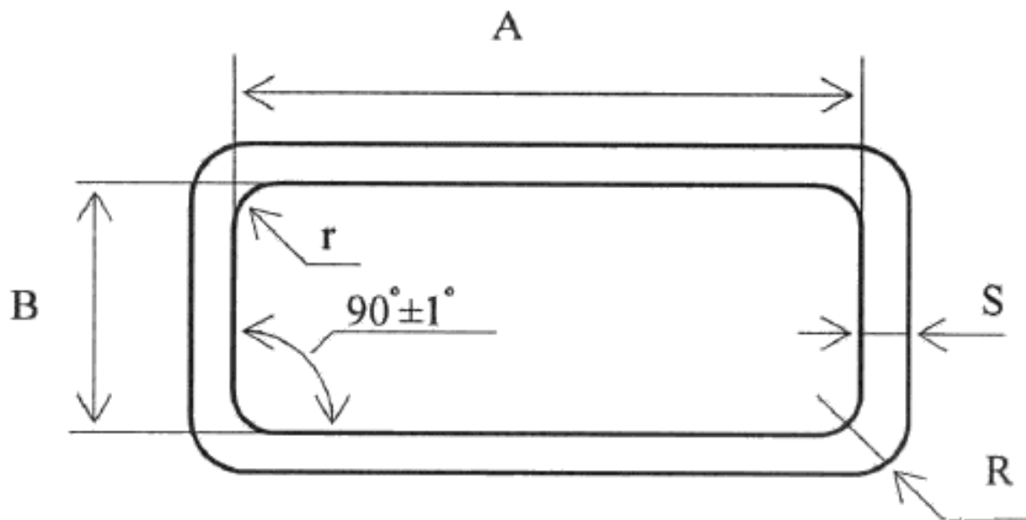
Рисунок 1 – Форма и геометрические размеры трубы
