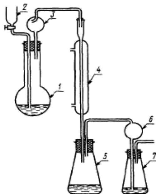
1 — колба для перегонки; 2 — капельная воронка; 3 — насадка Кельдаля; 4 — холодильник; 5 — приемник; 6 — трубка с расширением; 7 — контрольный приемник
